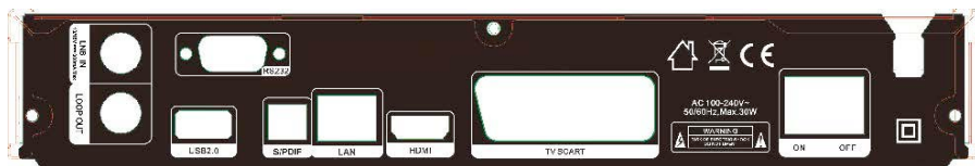
Obrázok 3. Zadný panel
