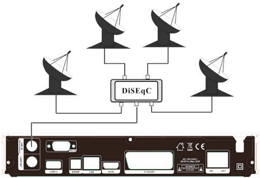
Obrázok 7. Pripojenie k LNB pomocou DiSEqC
